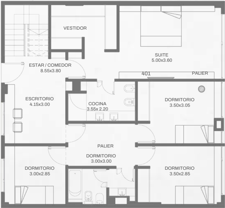
PLANTA BAJA
