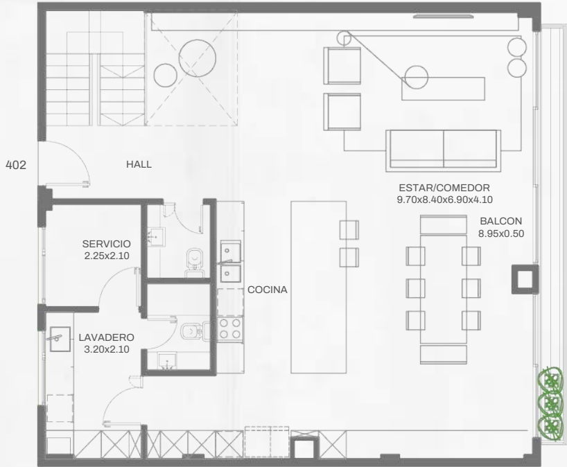
PLANTA ALTA
